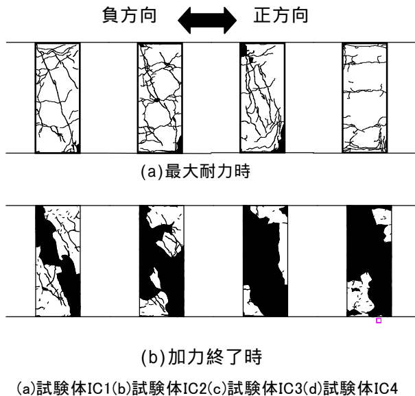
図-5 ひび割れ図
