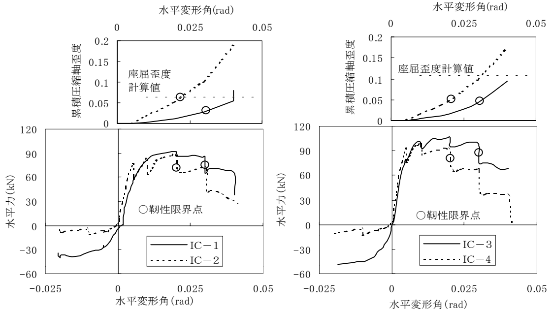
(a) \eta_{max}=0.32 (帯筋間隔50mm)の試験体
