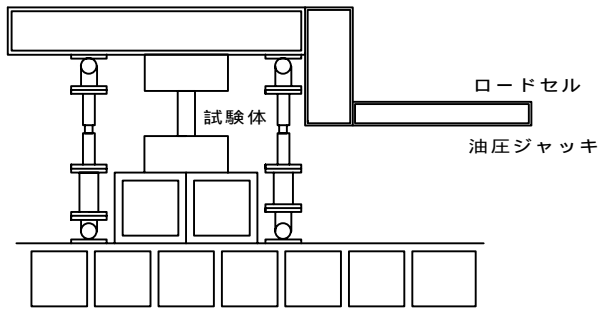
図-4 加力装置図
