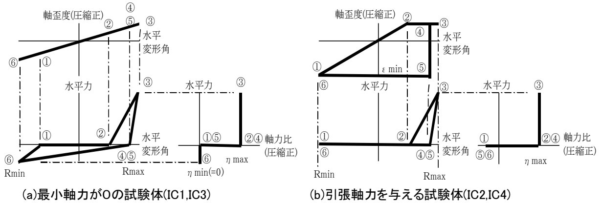
図-3 加力計画概念図
