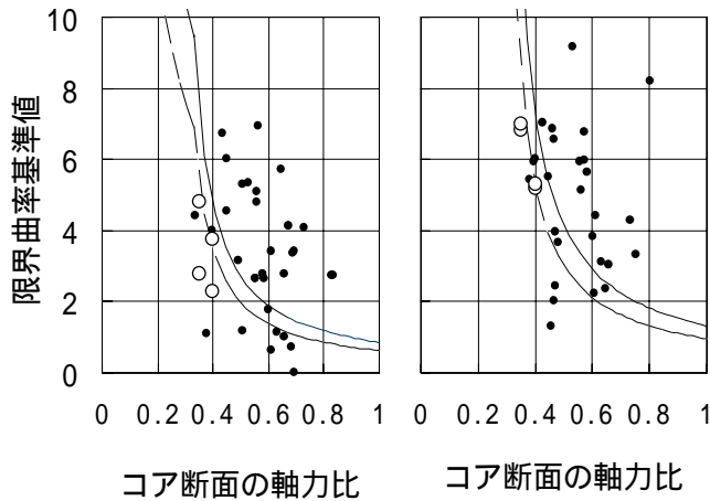
図-8 包絡線と主筋累積軸歪度の関係
