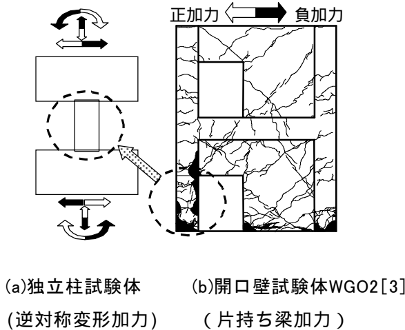
図-1 実験計画概念図
