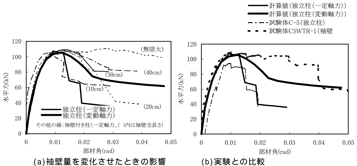
図-7 面外袖壁量の影響の検討
