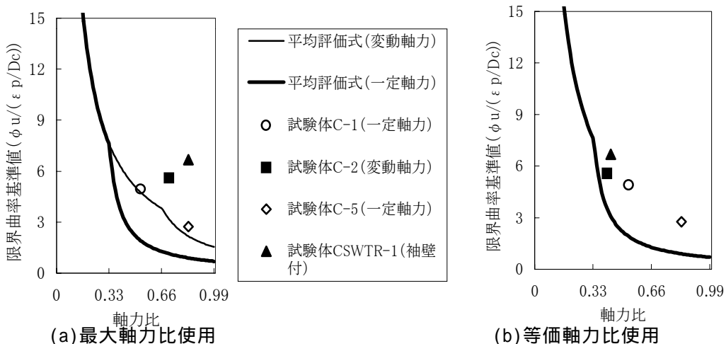
図-6 軸力比と変形能の関係の検討
