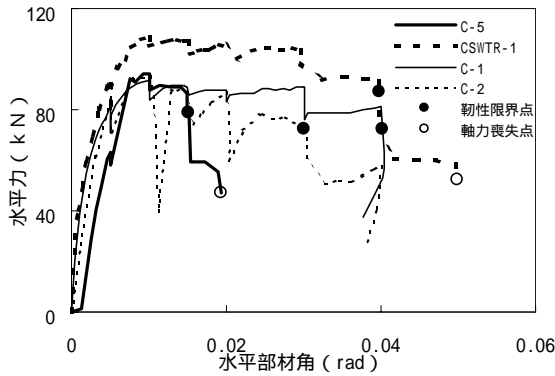
図-5 包絡線の比較（正方向）
