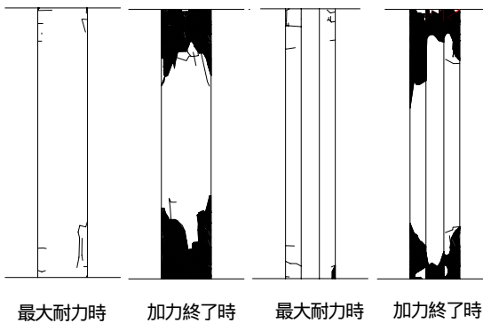
(a)C-5 (b)CSWTR-1 図-4 ひび割れ図
