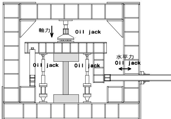
図-2 加力装置図
