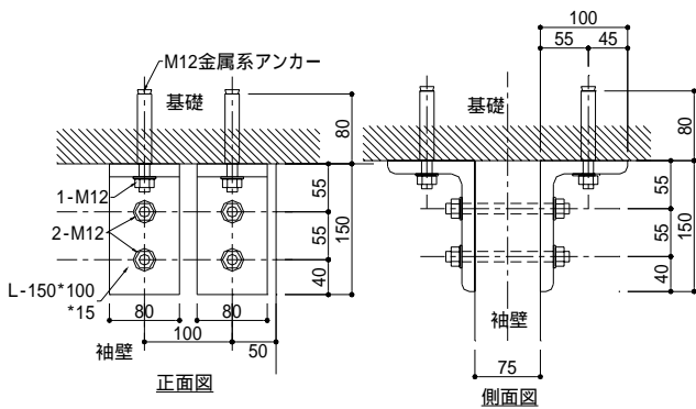
図 - 2 袖壁端部詳細図
